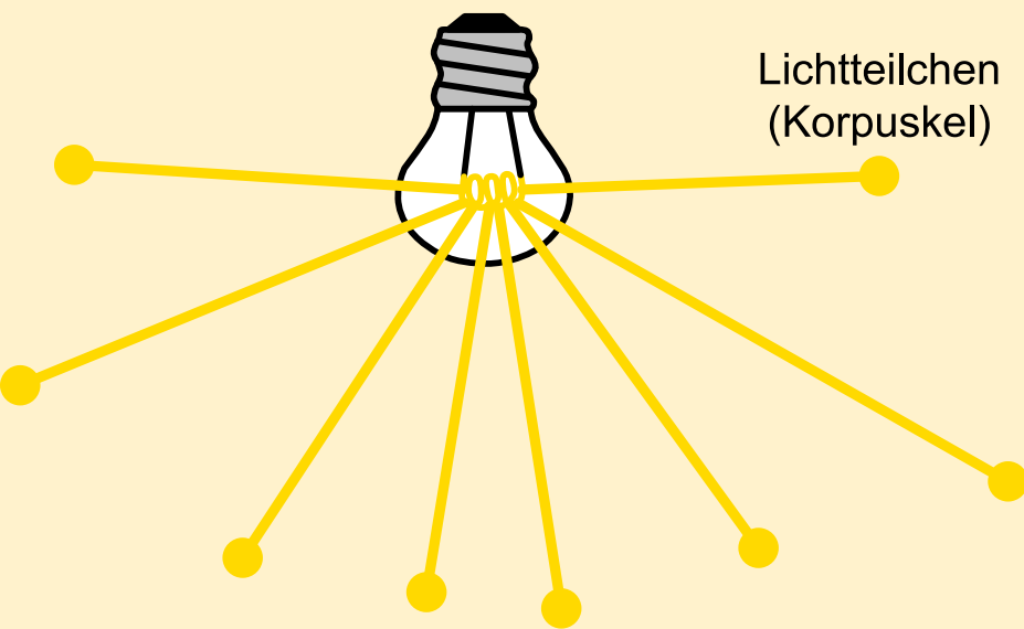
Geradlinige Lichtausbreitung
